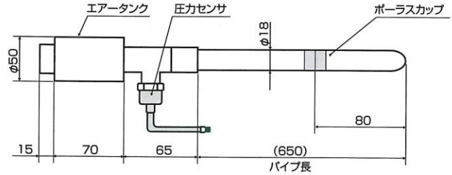
センサー部
